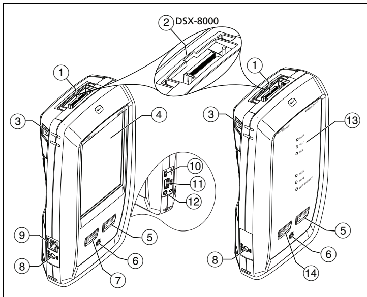
Abbildung 1. Anschlüsse, Tasten und LED-Anzeigen (Versiv 2 gezeigt)
