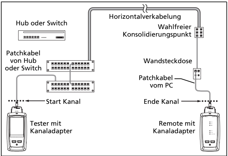
Abbildung 4. Kanal-Verbindungen für Verbindungen bis Cat 7 A
