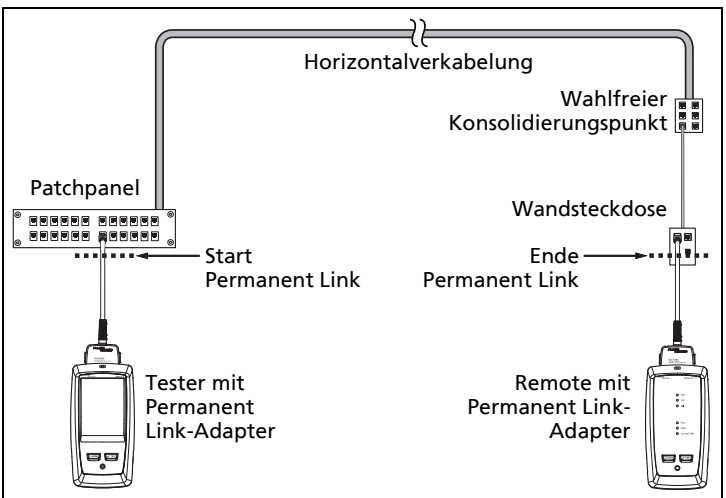
Abbildung 3. Permanent Link-Verbindungen für Verbindungen bis Cat 7 A
